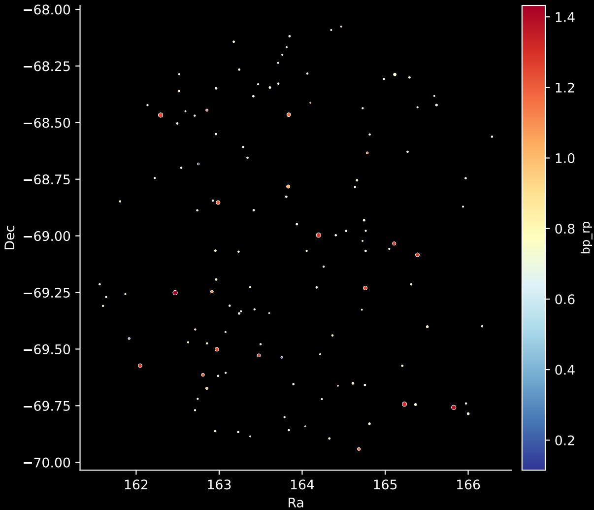
GALAH DR4 Field: [7208] Stars: 124
