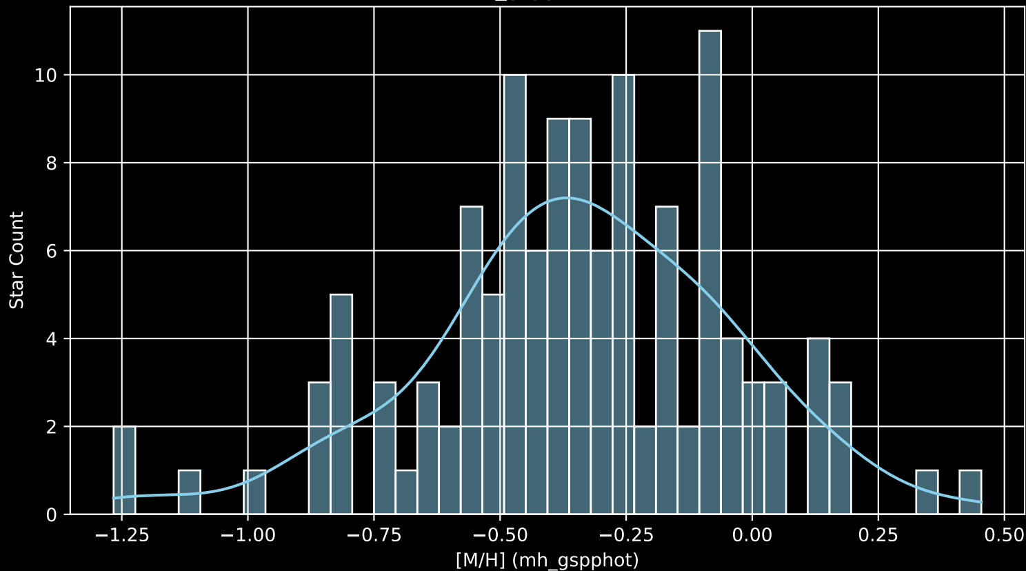
GALAH DR4 Field: [7208] [M/H] (mh_gspphot) (n= 124)
