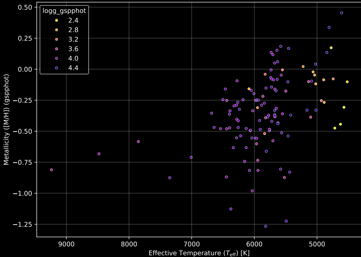
GALAH DR4 Field: [7208] Stellar Population Parameters (n= 124)
