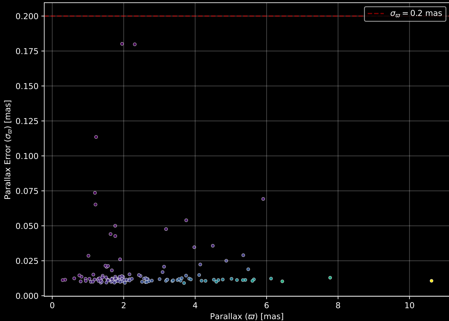
GALAH DR4 Field: [7208] Parallax Quality (n= 124)
